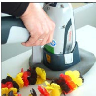
Röntgenfluoreszenzpistole Ermittlung von 30 Schwermetallen
